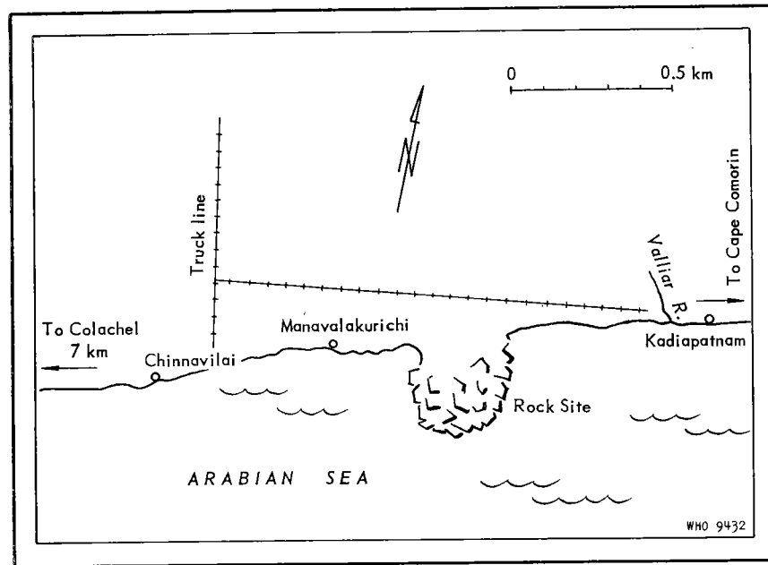
FIG. 3. THE MANAVALAKURICHI AREA
