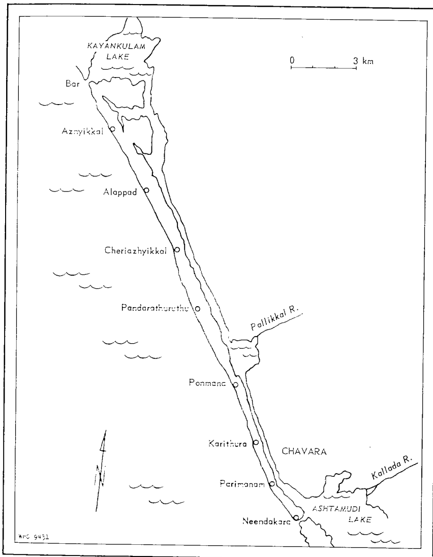
FIG. 2. THE CHAVARA-NEENDAKARA AREA
