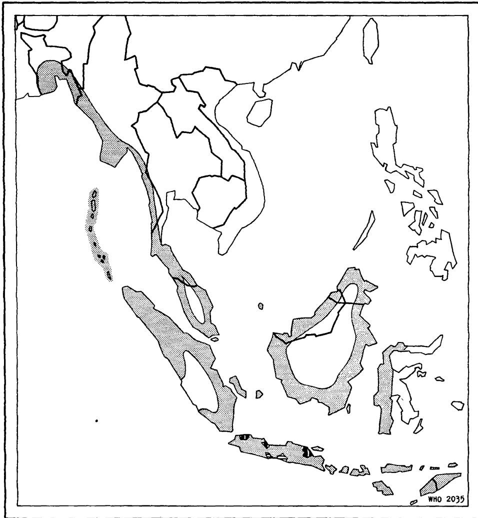
FIG. VI A. sundaiicus
