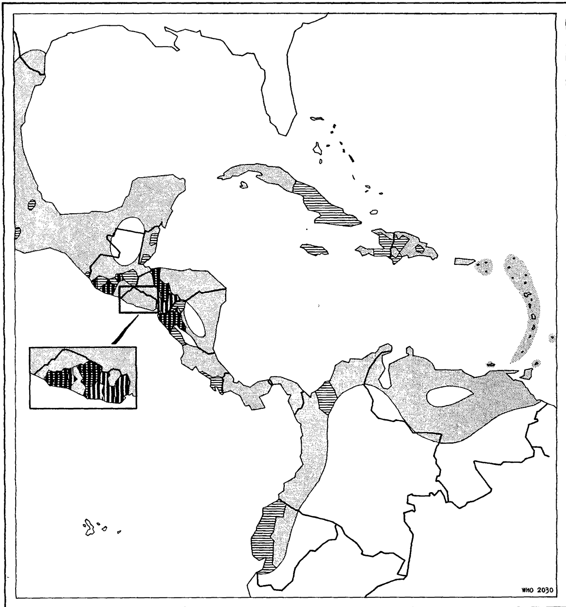
FIG. 1 A. albimanus
