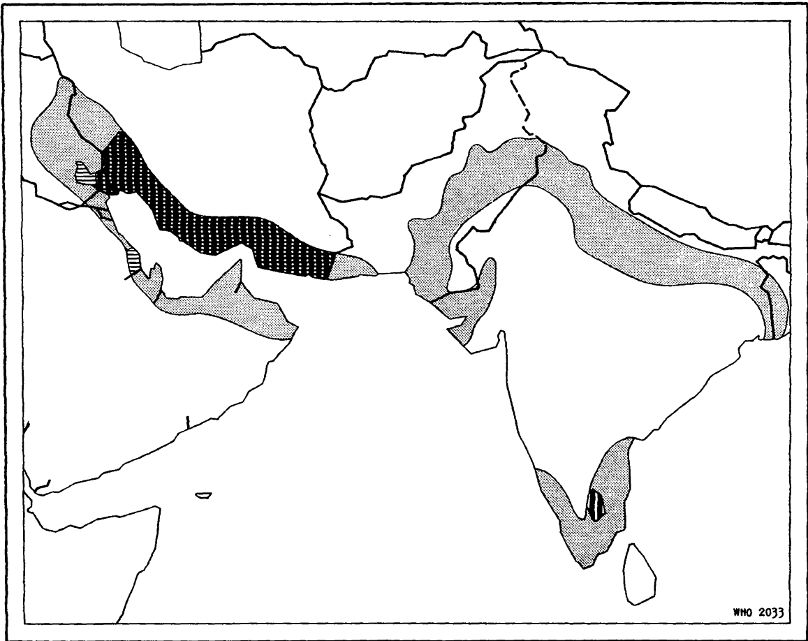
FIG. IV A. stephensi
