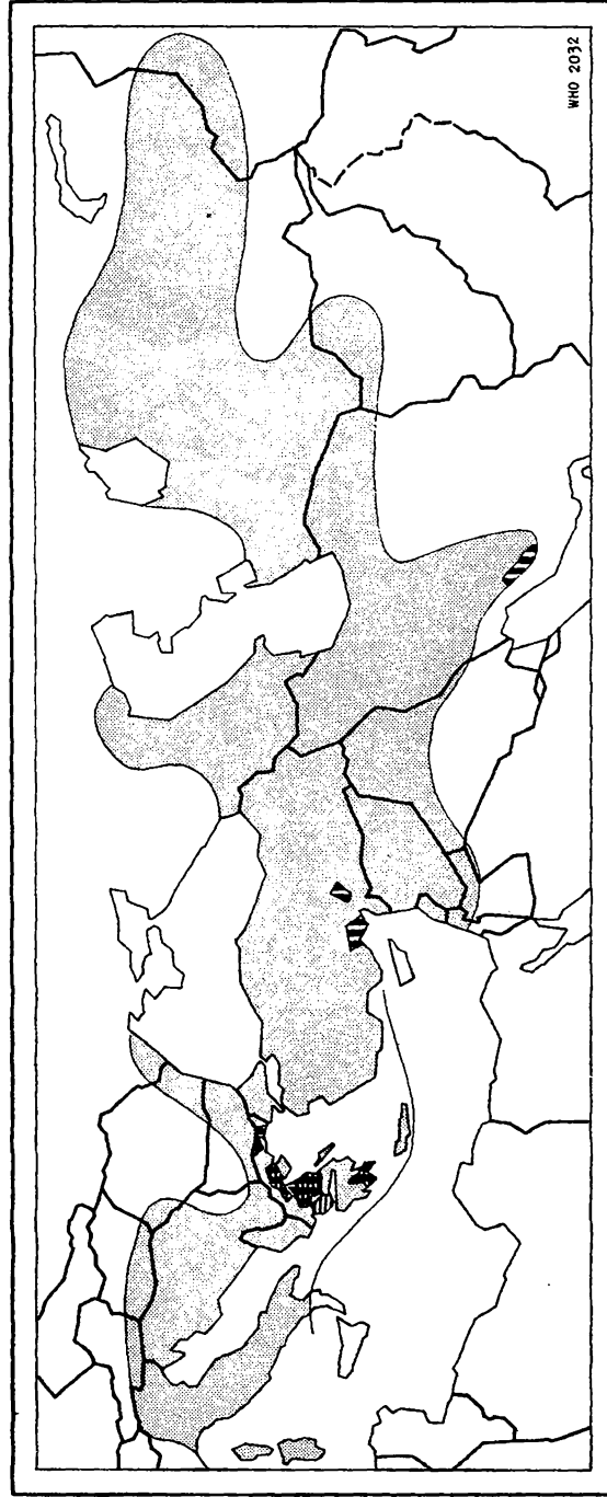
FIG. III A. sacharovi
