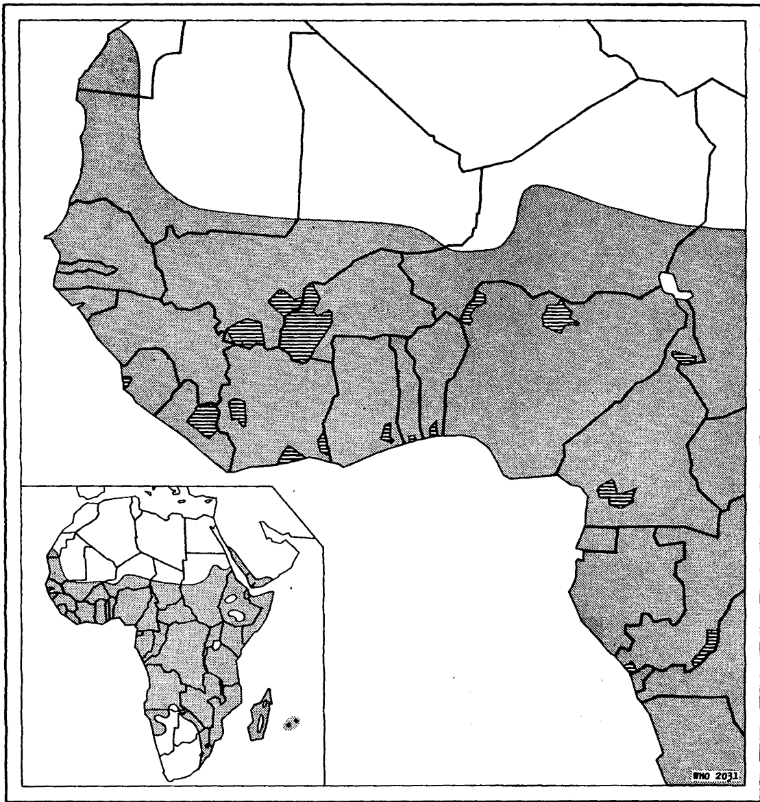
FIG. II A. gambiae
