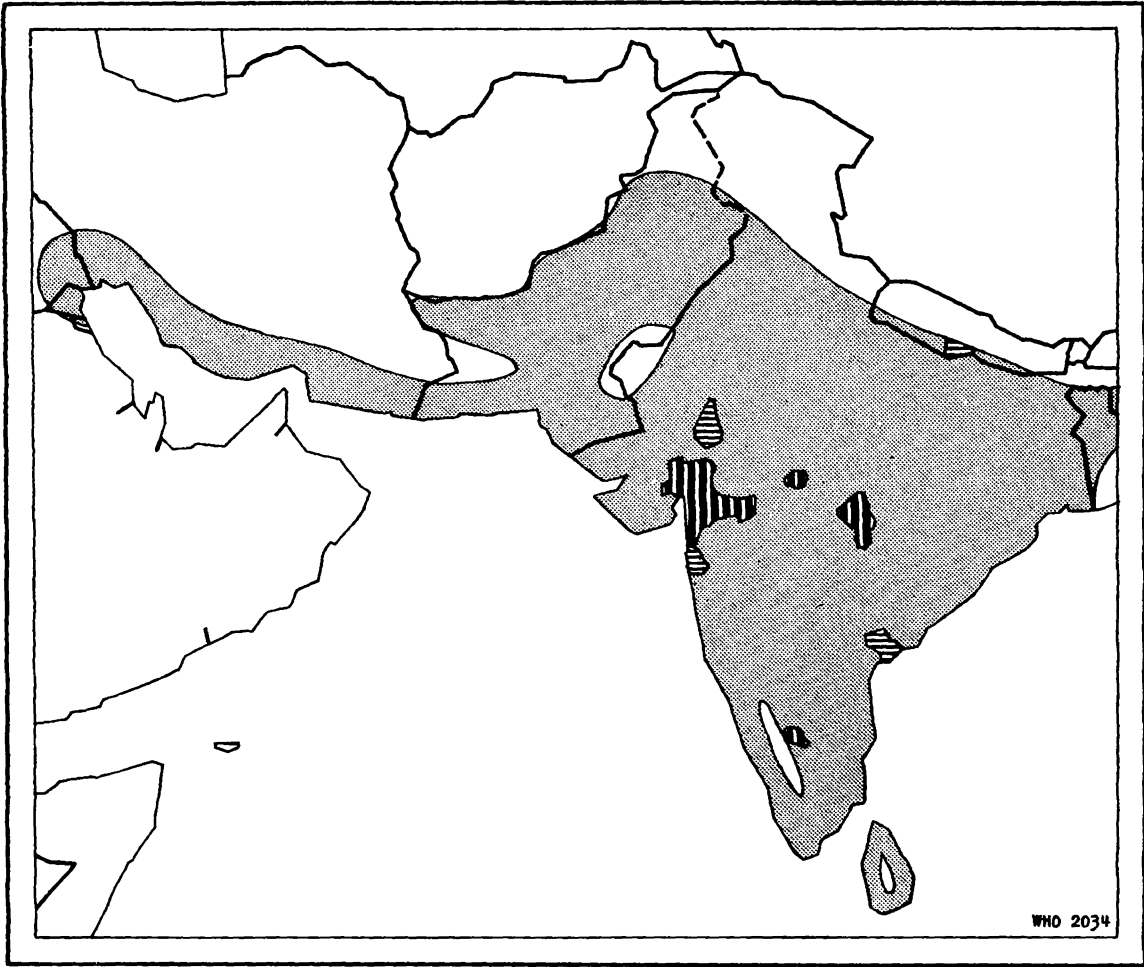
FIG. V A. culicifacies
